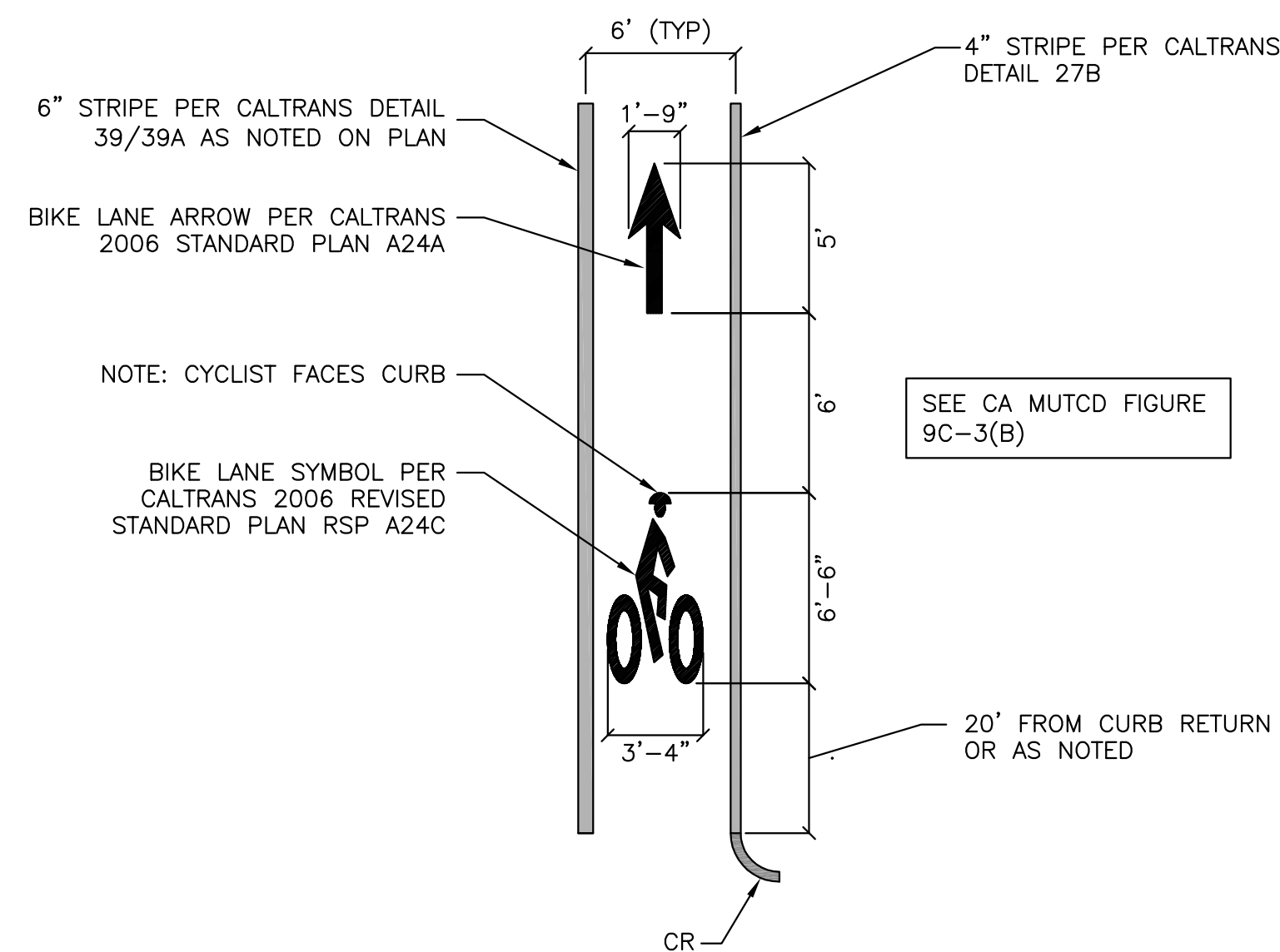
DETAIL 'B' BIKE LANE DETAIL N.T.S.
