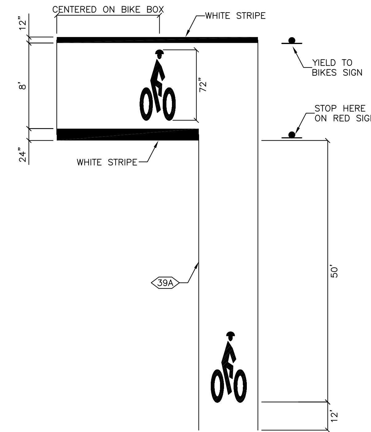
DETAIL 'D' BICYCLE BOX N.T.S.
